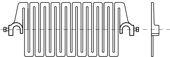
WG 9 0,045 Ω
